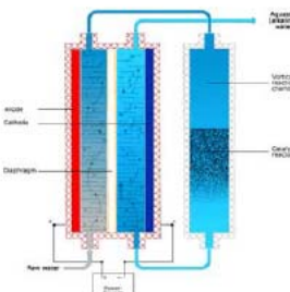
ESQUEMA DE PRINCIPIO
